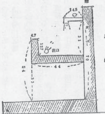
城東小学校の現施設
