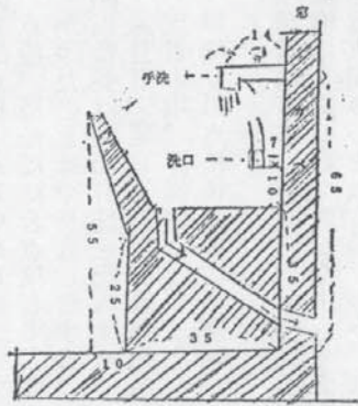
城東小学校の現施設
