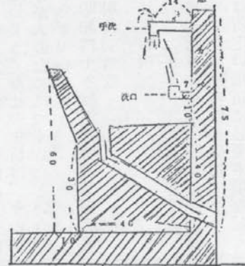
城東小学校の現施設(低学年) …各教室の出入口に近廊下窓側にある…
