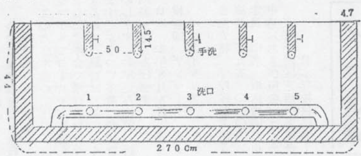
城東小学校の現施設
