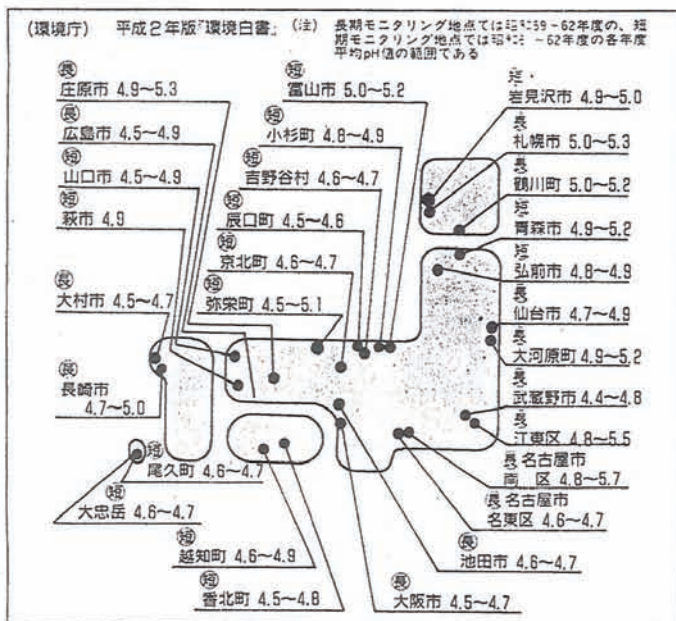
日本に降っている酸性雨
