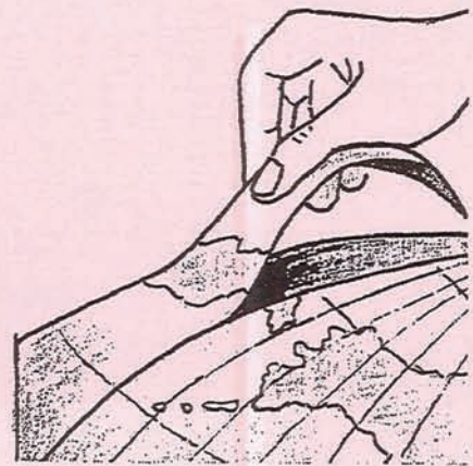
せいふつ こきゅう 生物が呼吸できる空気の層は、こんなに薄い
